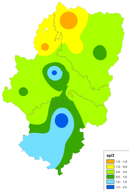
ÍNDICE DE PRECIPITACIÓN ESTANDARIZADO SEPTIEMBRE 2018 3 MESES
