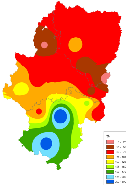
ANOMALÍA DE LA PRECIPITACIÓN SEPTIEMBRE 2018
