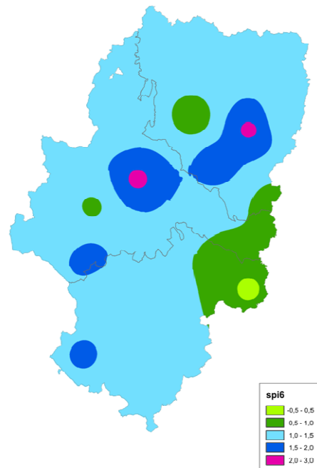
ÍNDICE DE PRECIPITACIÓN ESTANDARIZADO SEPTIEMBRE 2018 (6 MESES)
