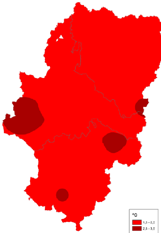
ANOMALÍA DE LA TEMPERATURA MEDIA SEPTIEMBRE 2018
