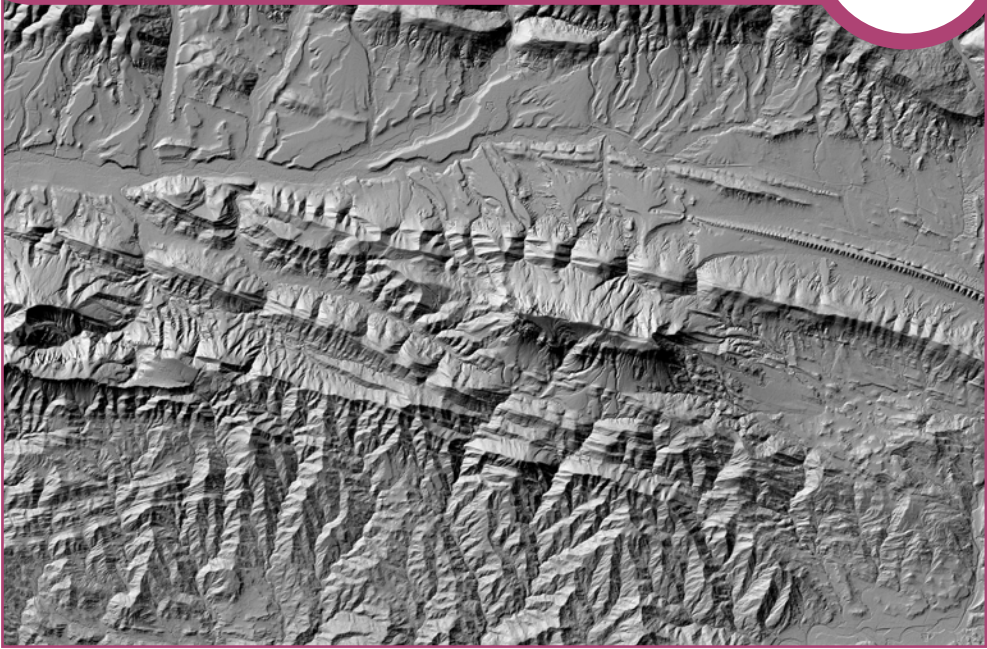
Detalle del Modelo Digital de Terreno (MDT) del entorno de Peña Oroel (Huesca). Año 2015
