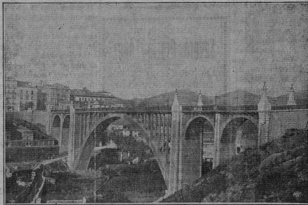
Admirable obra de Ingeniería, proyecto de don Fernando Hué, construcción de don Mariano Luña. Mide 34 metros de altura, y de sus cinco arcos, el central tiene 79 metros de luz o vano.
