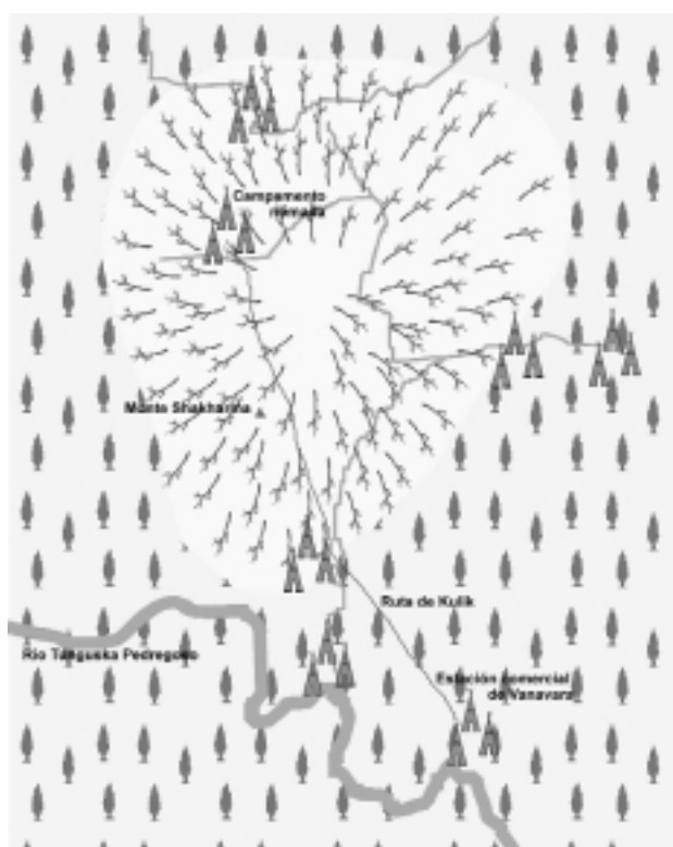
Mapa de la zona de Tunguska, basado en un dibujo publicado en la revista Cosmos . Imagen: G. Valentin.
