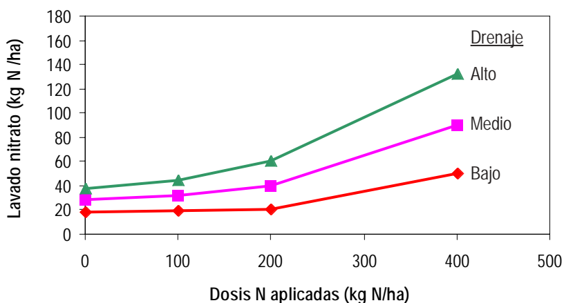
Figura 4. Efecto de la dosis de fertilizante N aplicado y del volumen de agua que drena por el perfil del suelo sobre la masa de N lixiviada en un cultivo de maíz (extraído de Pratt, 1984).
