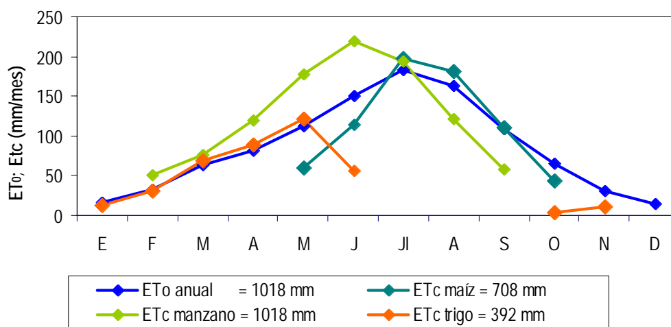
Figura 6. Evapotranspiración potencial ( ET_0 ) mensual del año medio y de distintos cultivos ( ETc ) en La Almunia de Doña Godina, Zaragoza (Martínez-Cob et al., 1998).
