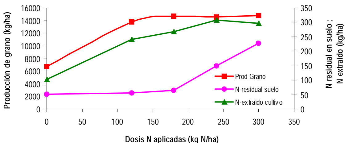
Figura 1. Efecto de la dosis de N sobre el rendimiento de grano de maíz, las extracciones de N del cultivo, y el N residual en el suelo (0-120 cm) después del cultivo. Datos procedentes de un ensayo en la finca experimental de Montañana del C.I.T.A. (Gobierno de Aragón).
