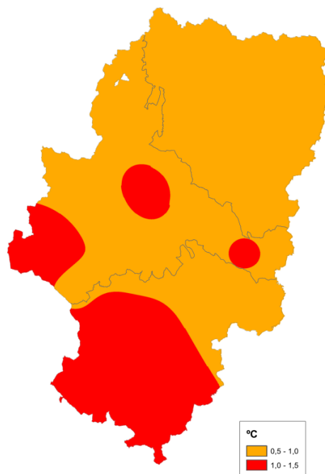
ANOMALÍA DE LA TEMPERATURA MEDIA AÑO 2017
