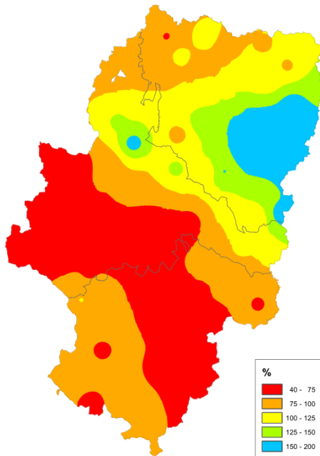
ANOMALÍA (%) DE LA PRECIPITACIÓN PRIMAVERA 2017
