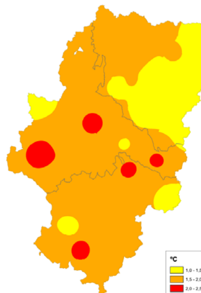
ANOMALÍA TEMPERATURA MEDIA PRIMAVERA 2017
