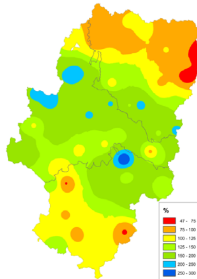
ANOMALÍA (%) DE LA PRECIPITACIÓN VERANO 2017
