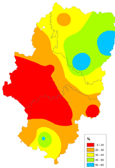
ANOMALÍA (%) DE LA PRECIPITACIÓN OTOÑO 2017
