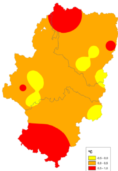
ANOMALÍA DE LA TEMPERATURA MEDIA OTOÑO 2017
