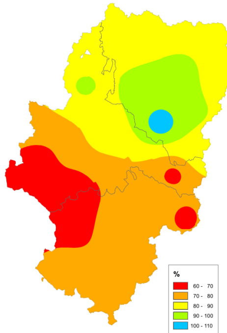
ANOMALÍA (%) DE LA PRECIPITACIÓN AÑO 2017
