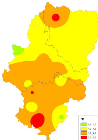
ANOMALÍA TEMPERATURA MEDIA VERANO 2017
