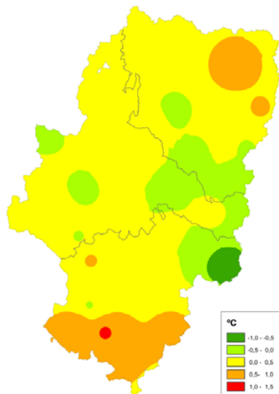
ANOMALÍA TEMPERATURA MEDIA INVIERNO 2016-2017
