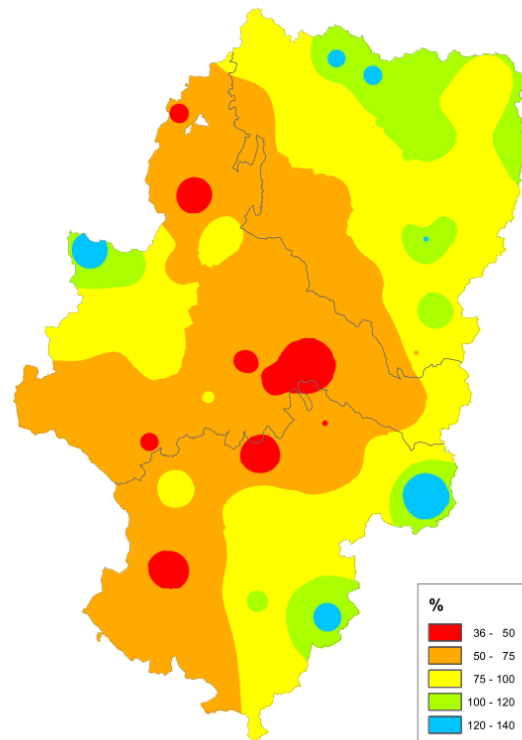
ANOMALÍA (%) DE LA PRECIPITACIÓN INVIERNO 2016-2017
