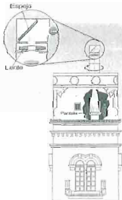
Croquis del funcionamiento de una cámara oscura.
