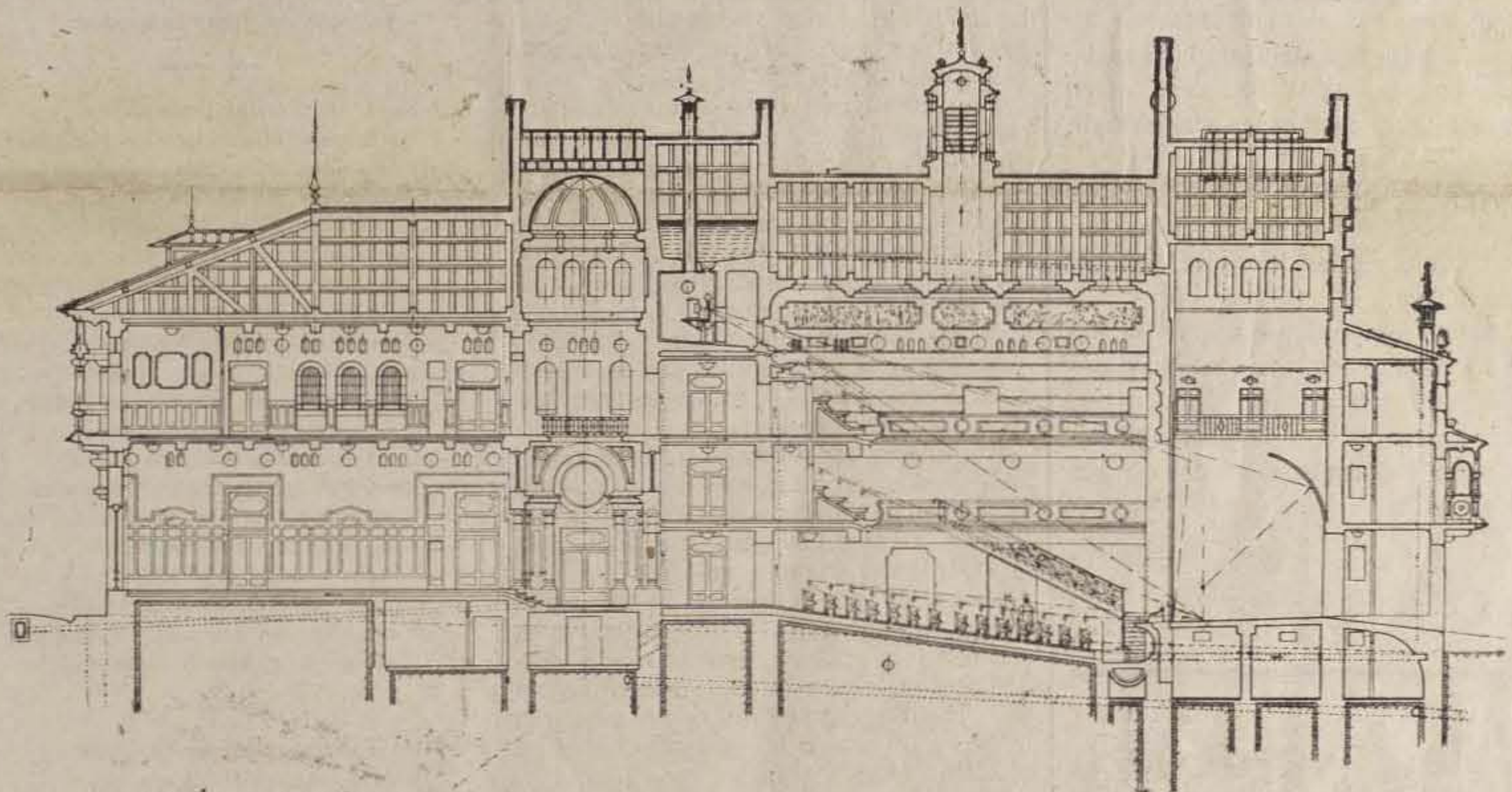
SECCIÓN LONGITUDINAL
