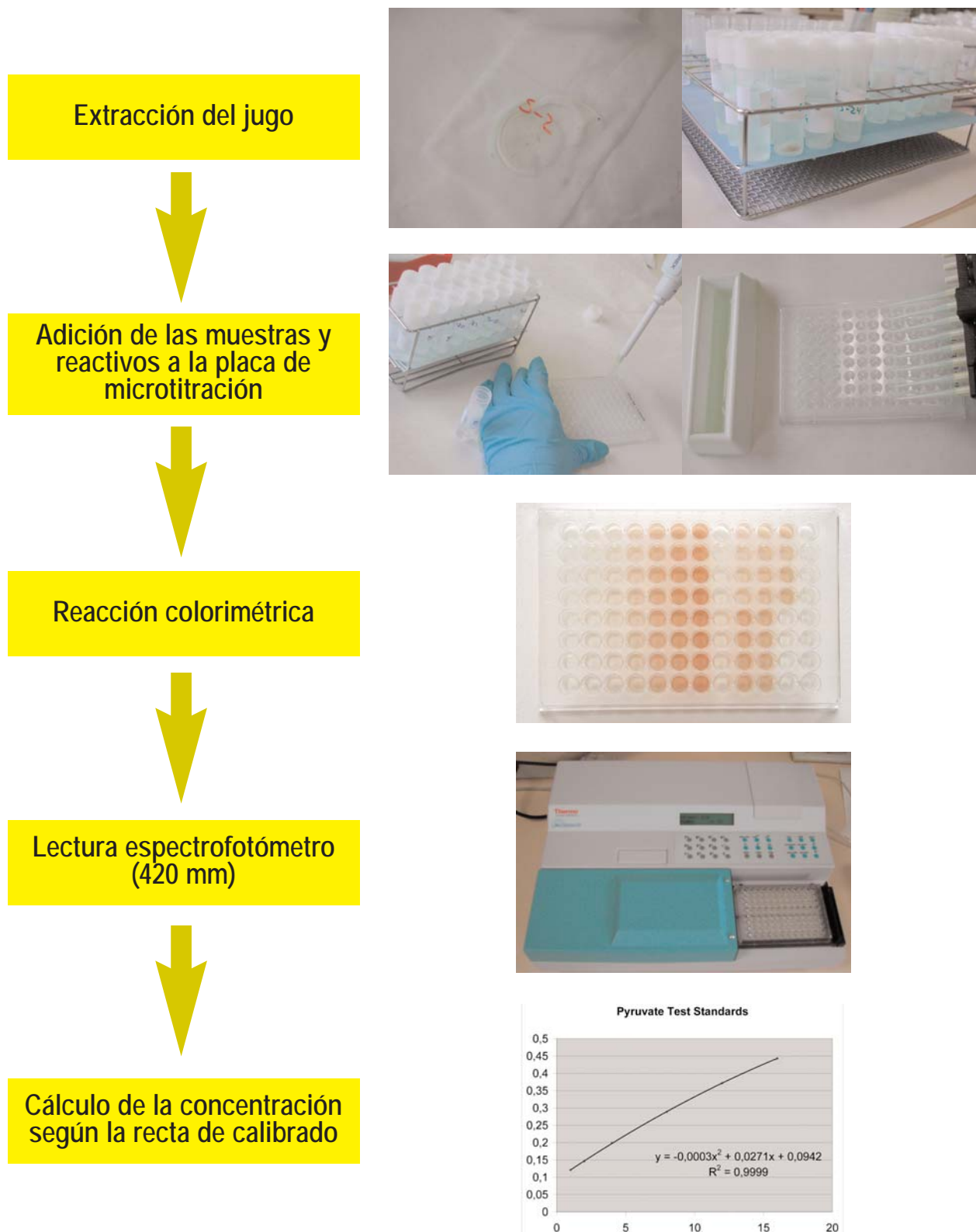
Fig. 4: Metodología para la cuantificación del contenido en ácido pirúvico de las muestras de cebolla.
